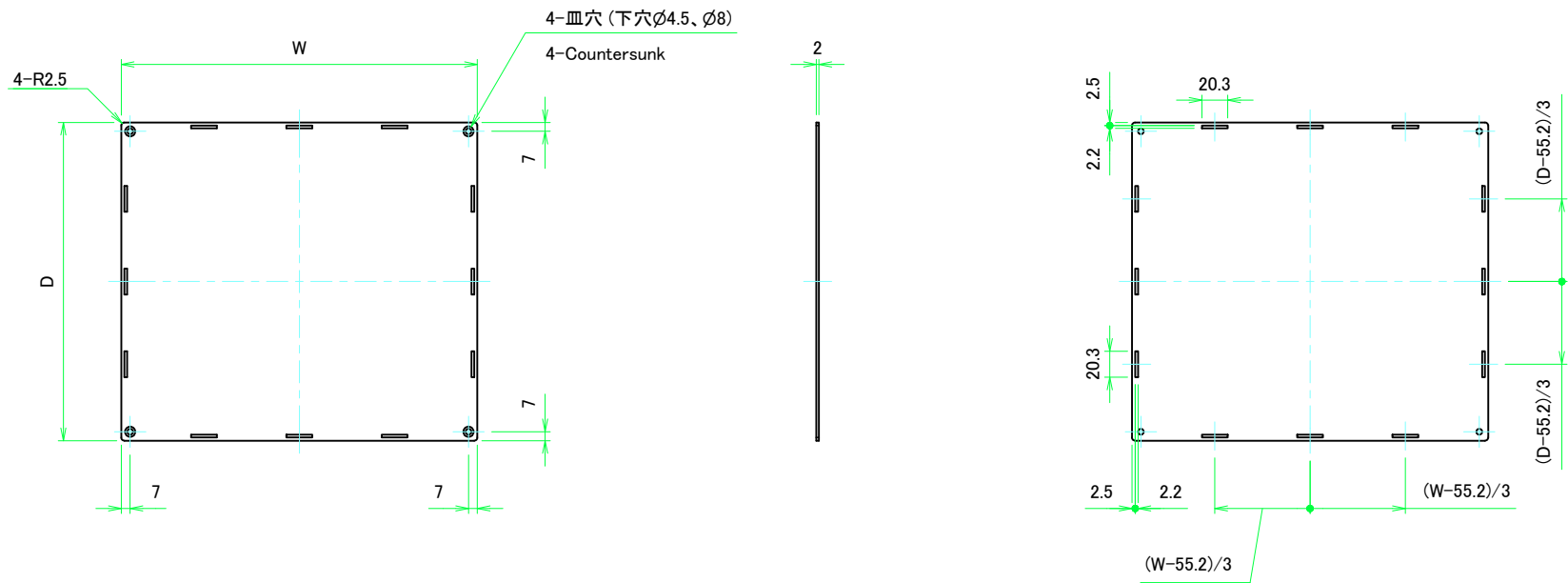
上カバー裏面 / Top cover Backside
