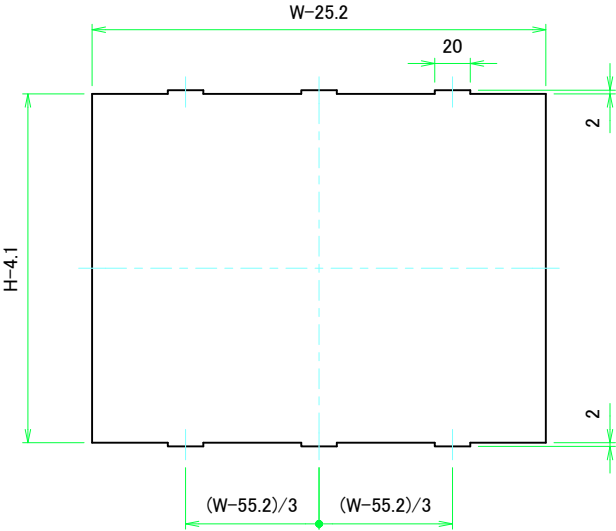
Wパネル1表面 / W Panel 1 Frontside
