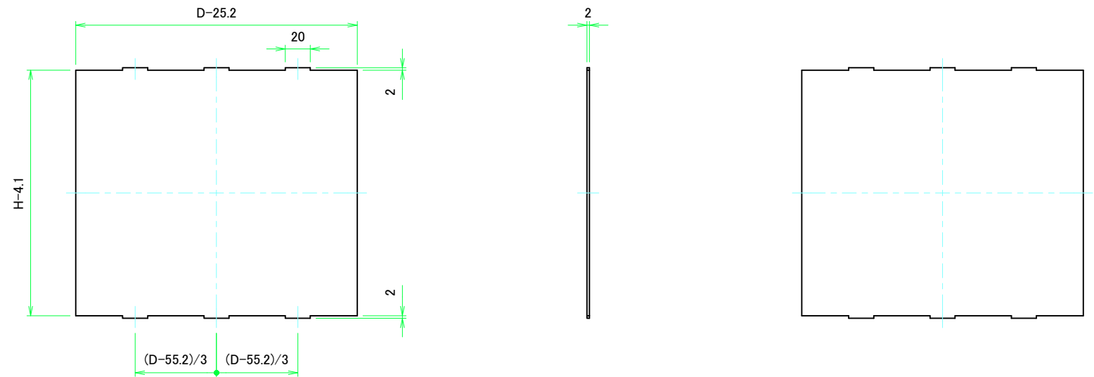
Dパネル1表面 / D Panel 1 Frontside
